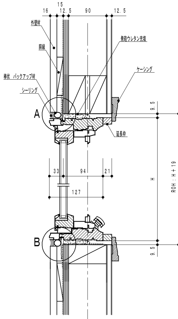
縦断面図
