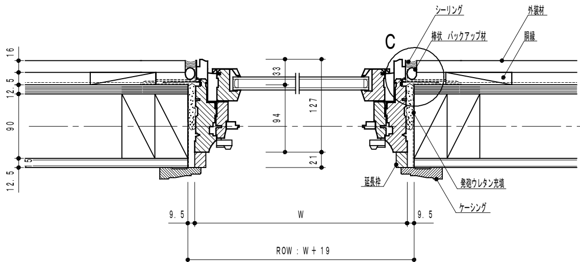
横断面図
