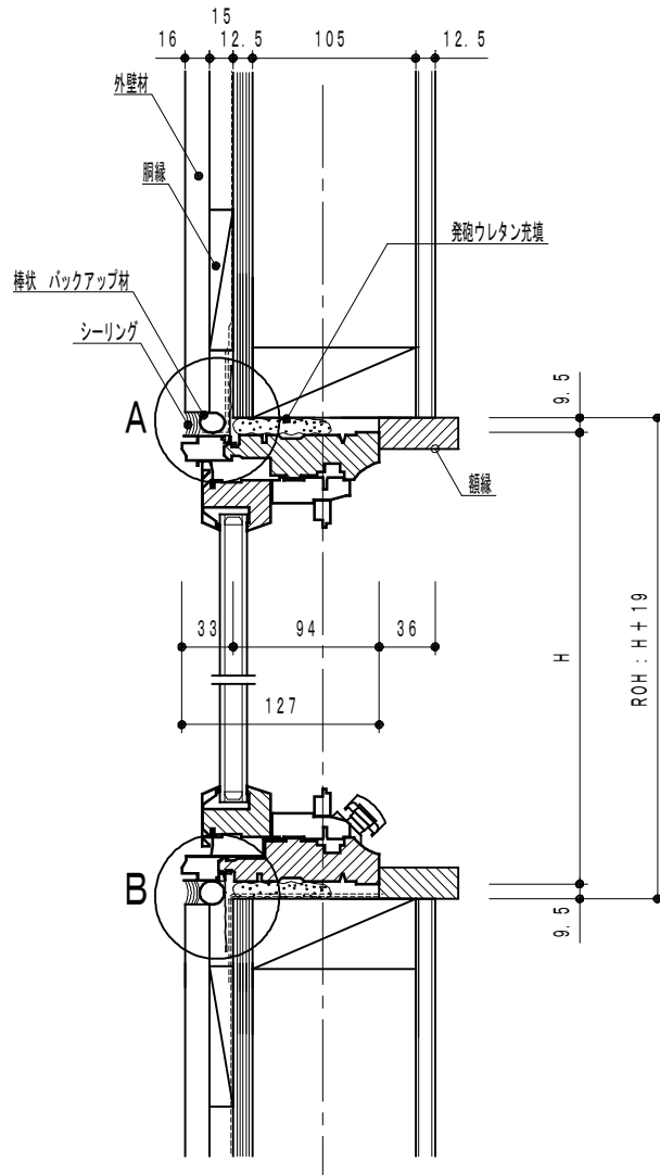
縦断面図
