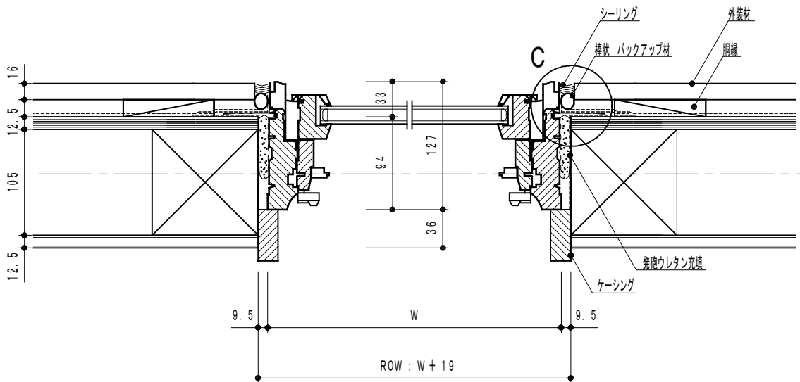
横断面図
