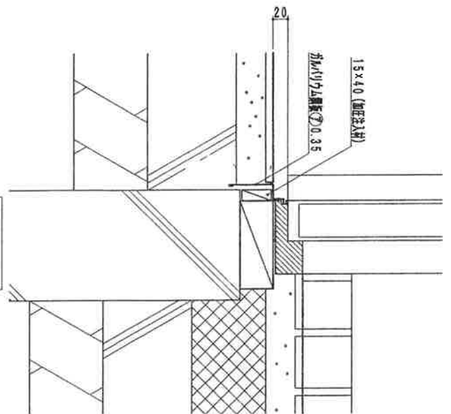
A部詳細
