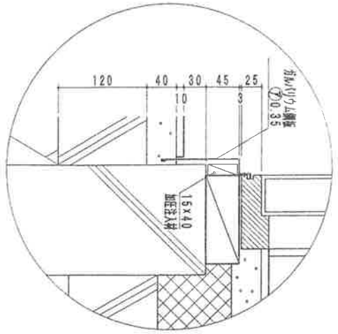
A部詳細
