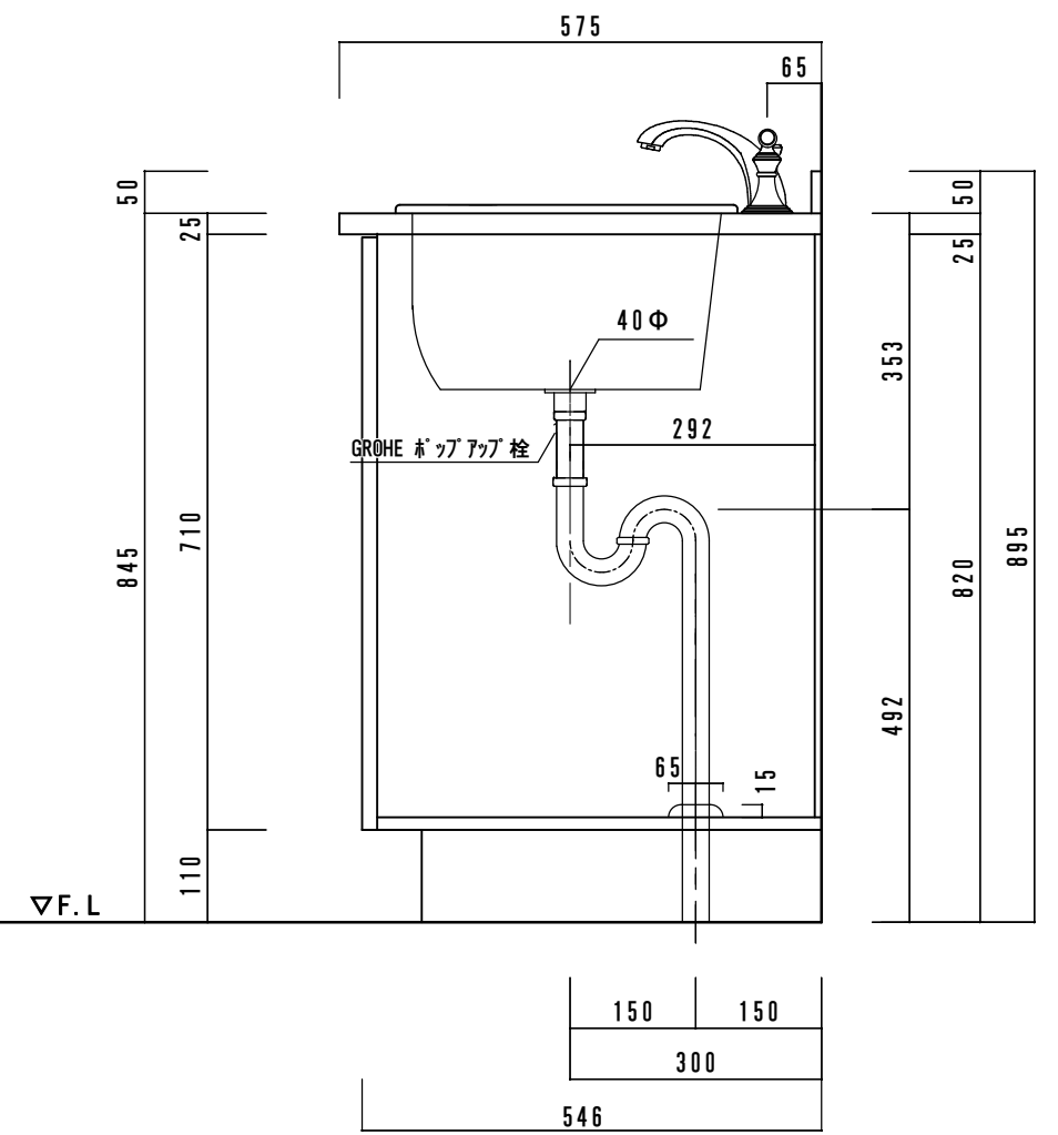
アクリル人工大理石断面図
