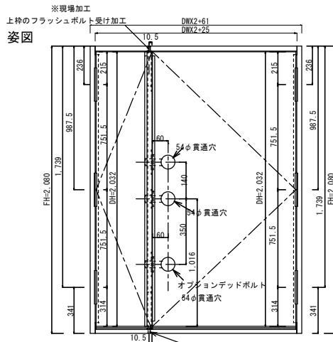
HOWDY 玄関ドア納まり図
