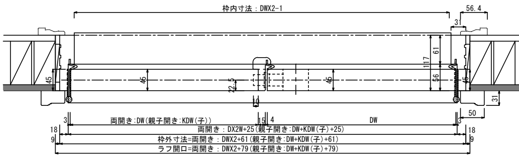
※現場加工 上枠のフラッシュボルト受け加工
