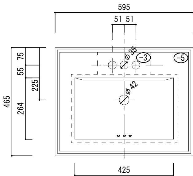
上面図
