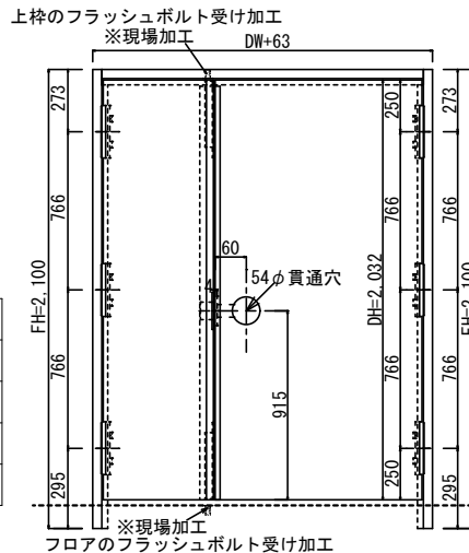
HOWDY 内部ドア納まり図
