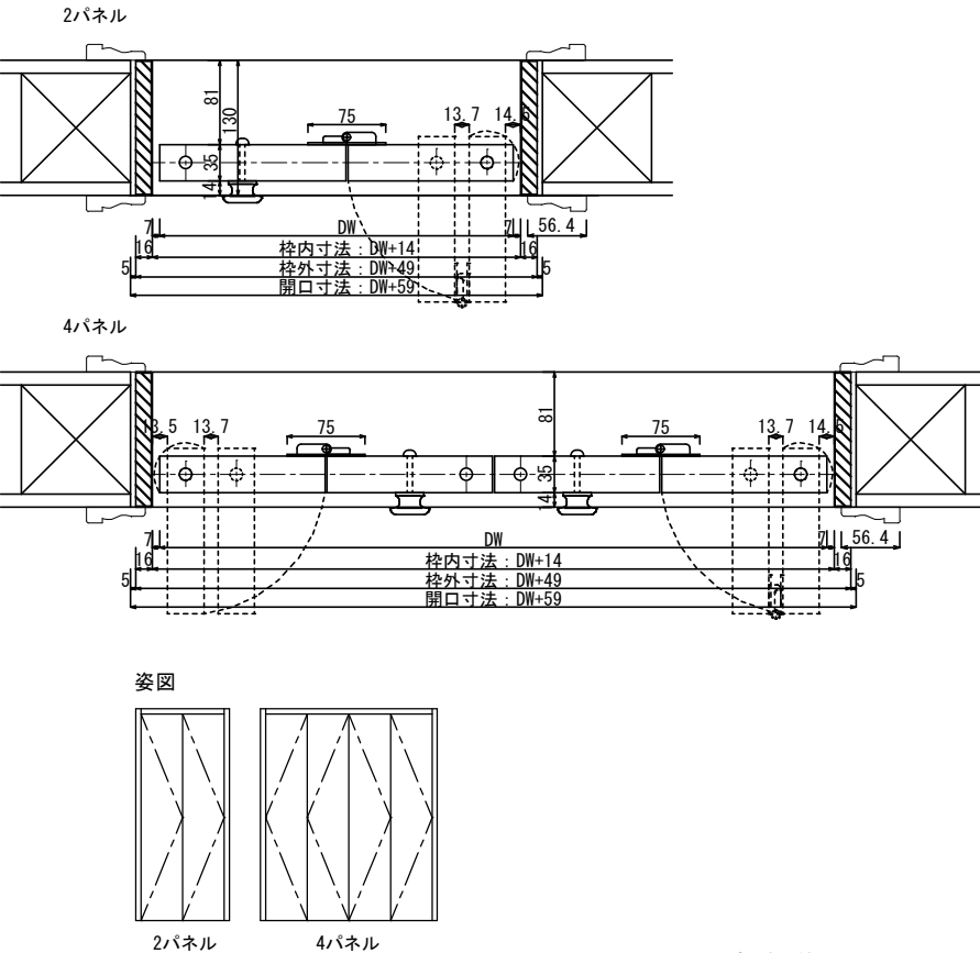
HOWDY 内部ドア納まり図
