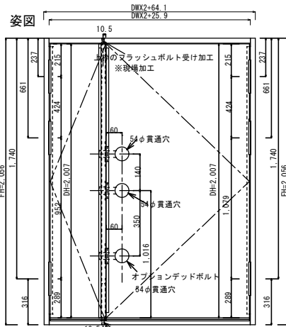
HOWDY 玄関ドア納まり図
