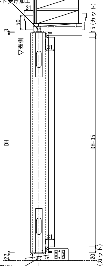
※現場加工 ボトムシルのフラッシュボルト受け加工
