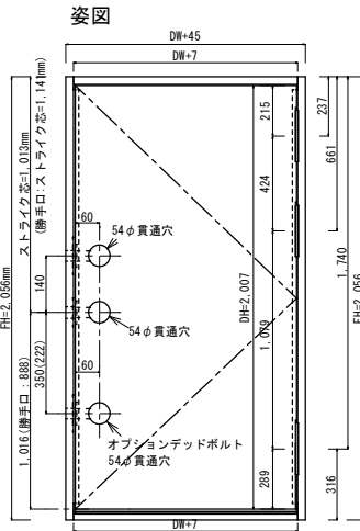
HOWDY 玄関ドア納まり図
