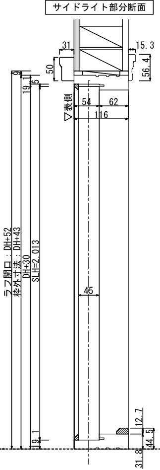
サイドライト部分断面
