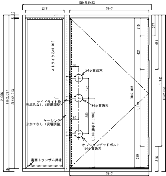
姿図
