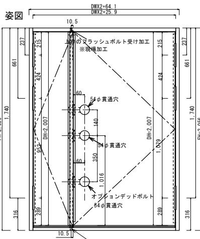
HOWDY 玄関ドア納まり図
