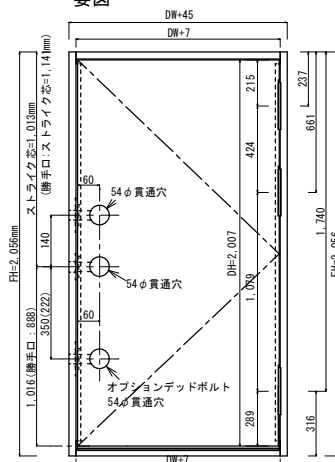
HOWDY 玄関ドア納まり図
