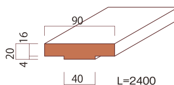
縦モール材
