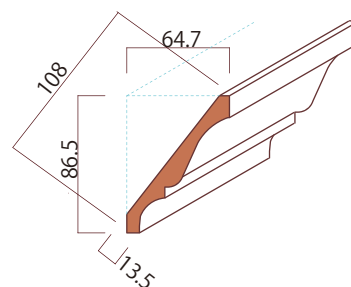
廻り縁
