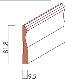
巾木
