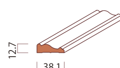
HM-H3005-7 へム
