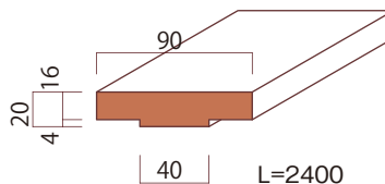
TW-9016T-24 レッドオーク(単板貼)
