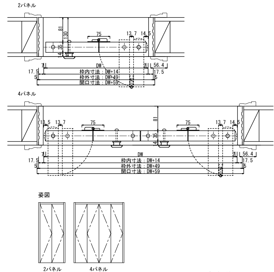
HOWDY 内部ドア納まり図
