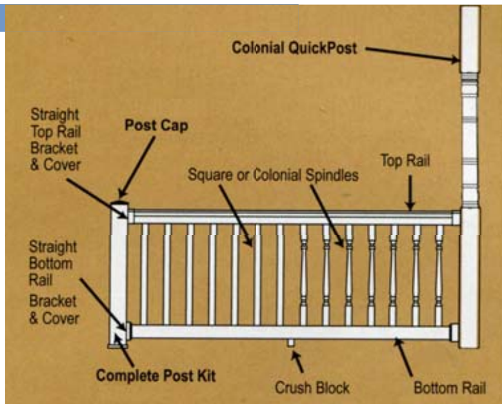
コロニアル・クイックポスト 専用トリムキット (上下セット)
