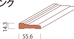
HM-H3004A ヘム 7F 55.6×14.3×2134 ¥3,700 12F 55.6×14.3×3657 ¥6,600
