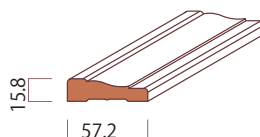
HM-WM356 ヘム 7F 57.2×15.8×2134 ¥3,600 12F 57.2×15.8×3657 ¥7,100
